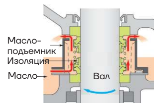
Направление вращения
