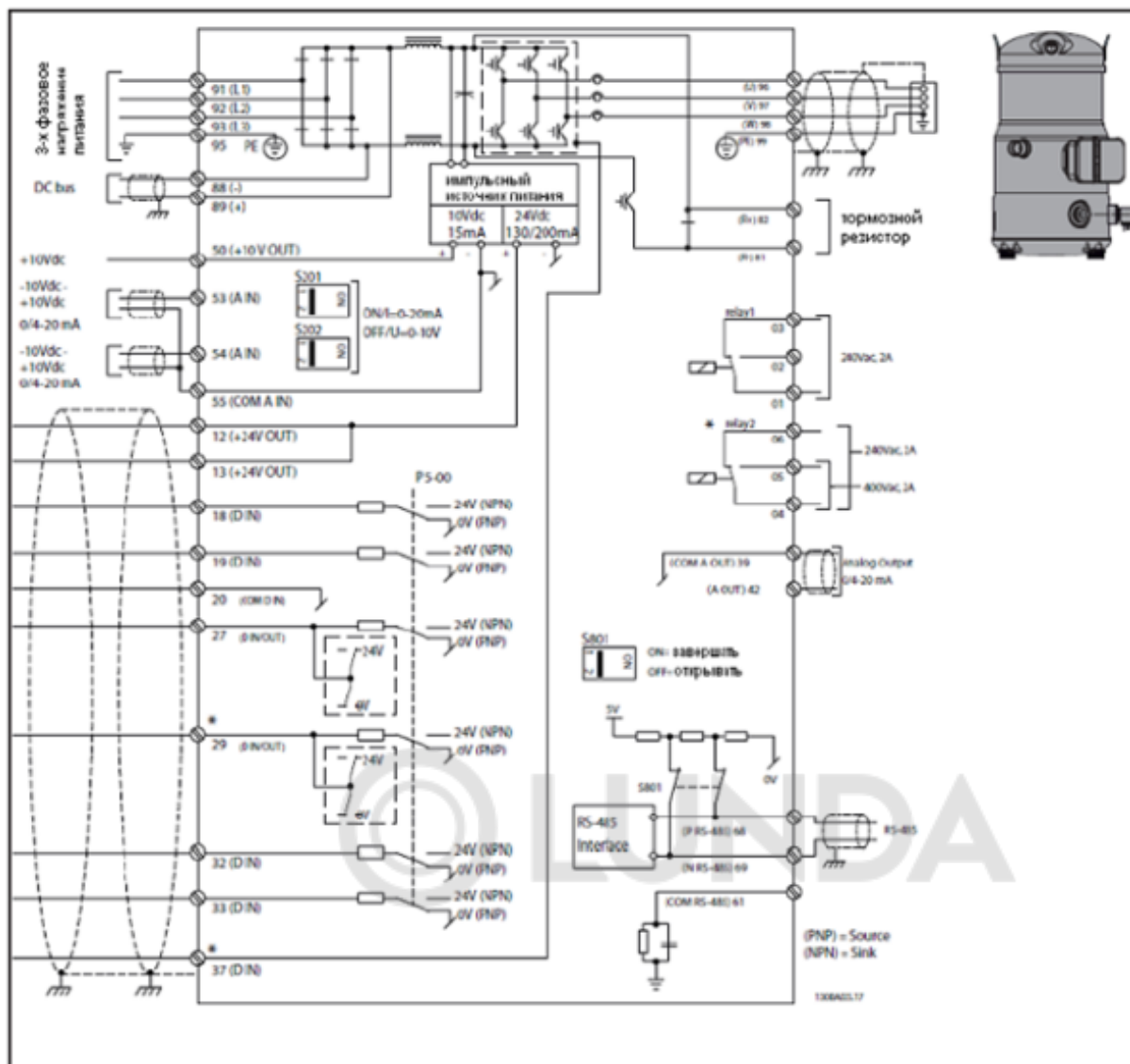
Схема подключения
