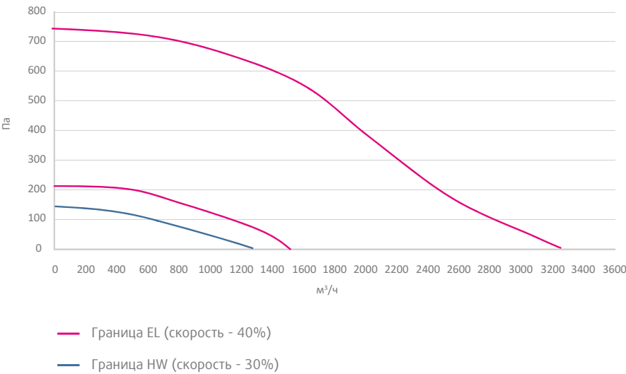
График производительности Torvex SF08
