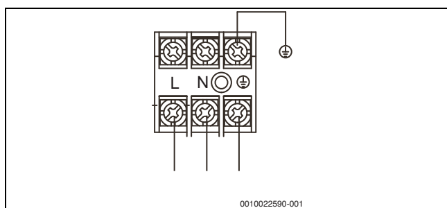
Рис. 39 Входное питание
