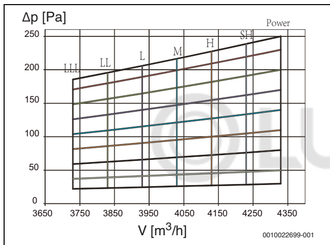
Рис. 31 AF-DH 250-1
