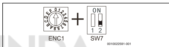
Рис. 46 ENC1 + SW7_2
