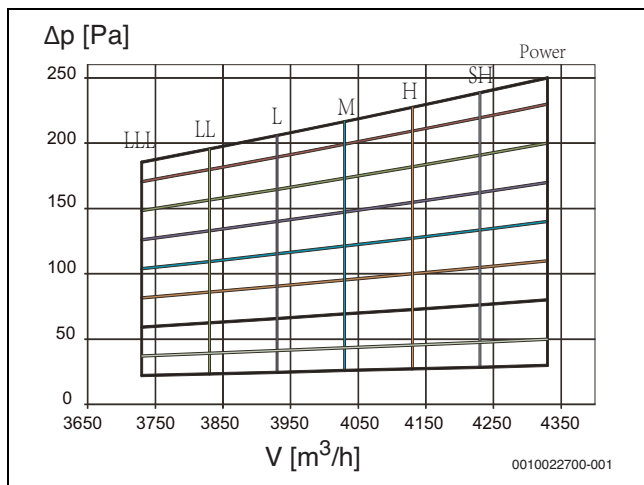
Рис. 32 AF-DH 280-1
