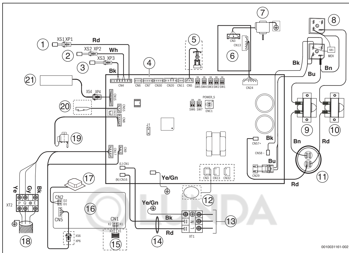
Рис. 53 Электропроводка, прототип 200–280
