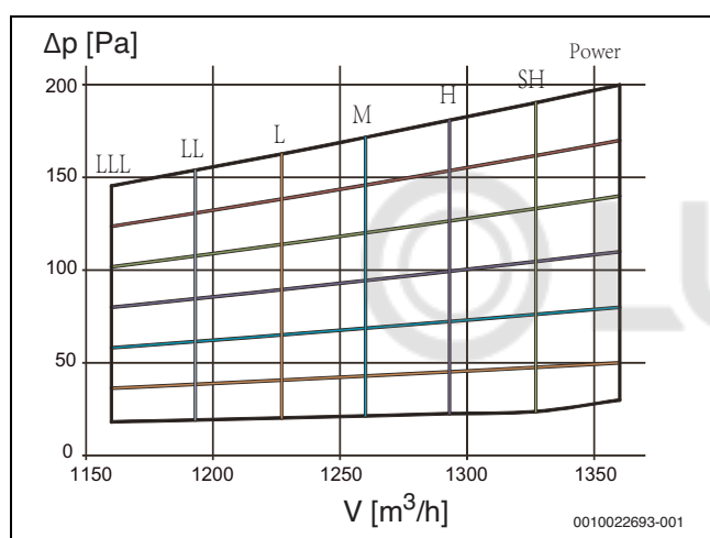
Рис. 25 AF-DH 80-1
