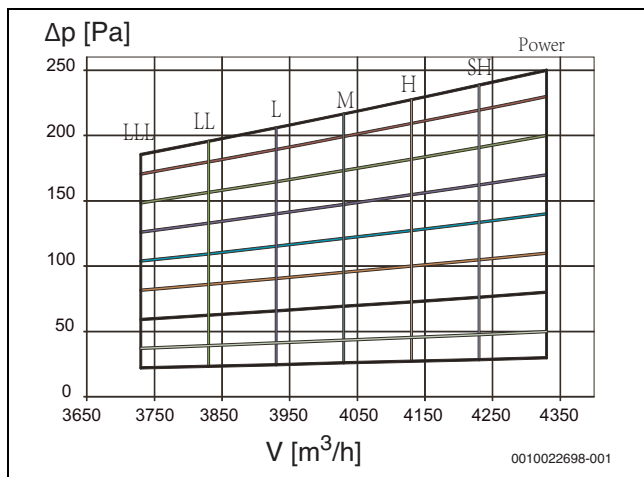
Рис. 30 AF-DH 200-1
