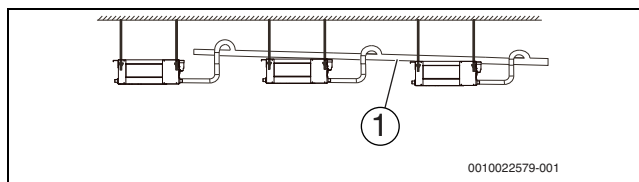
Рис. 20 Монтаж сливного трубопровода с водяным насосом
