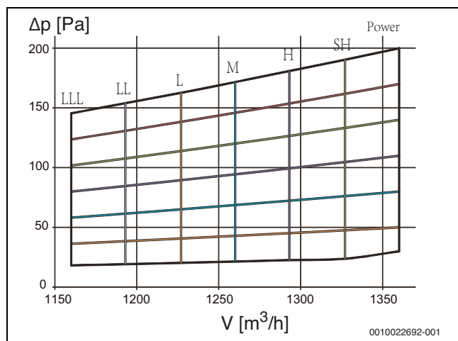
Рис. 24 AF-DH 71-1
