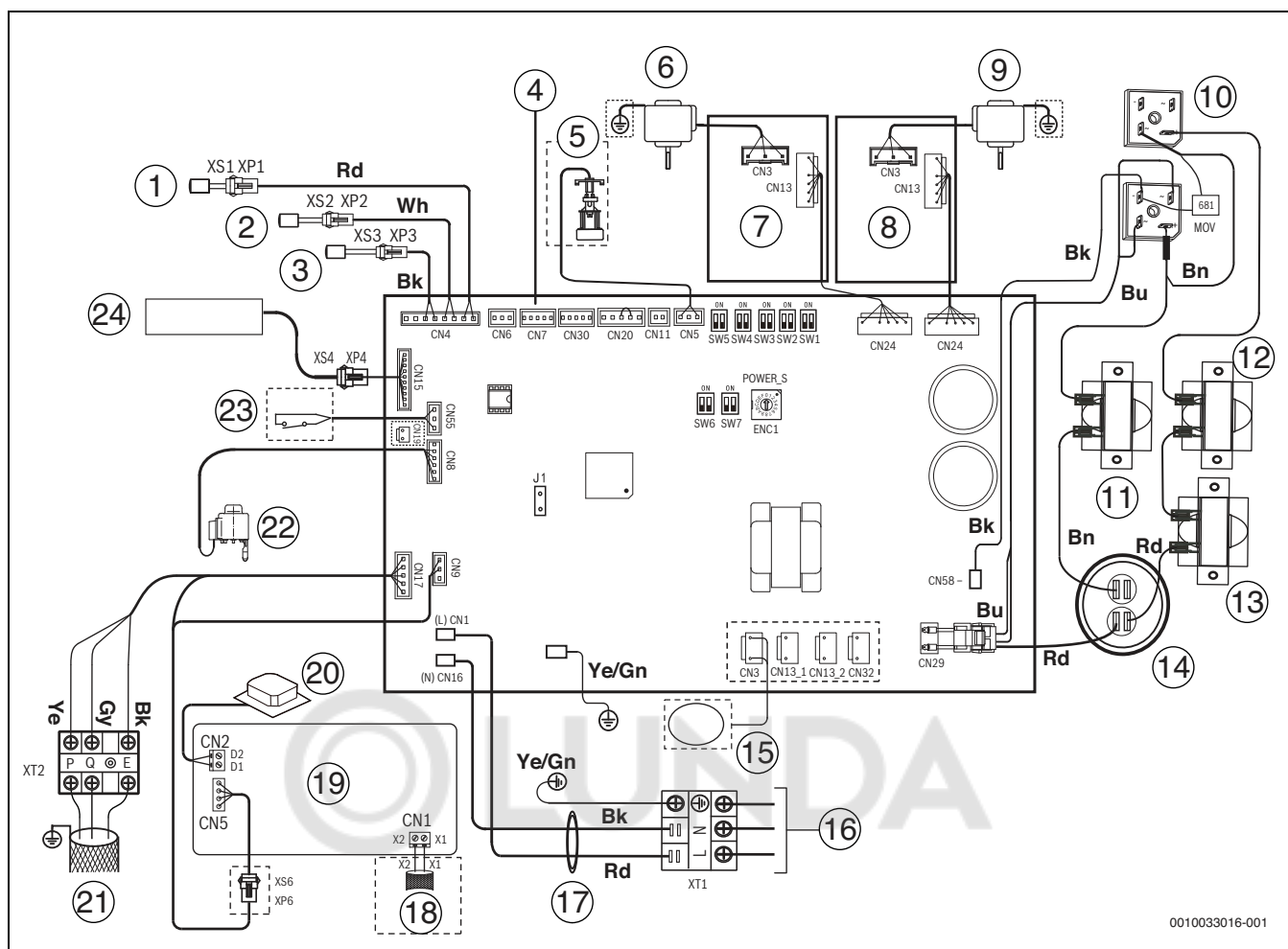
Рис. 54 Электропроводка, прототип 400–560
