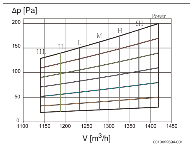
Рис. 26 AF-DH 90-1
