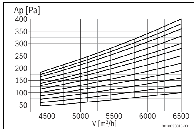
Рис. 33 AF-DH 400-1, AF-DH 450-1
