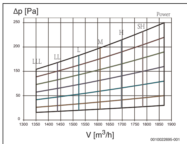
Рис. 27 AF-DH 112-1
