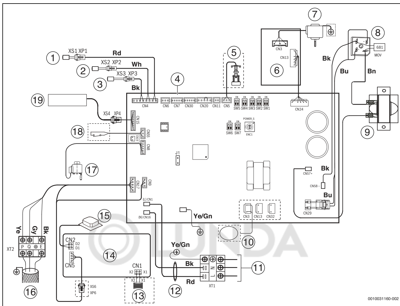
Рис. 52 Электропроводка, прототип 90–160
