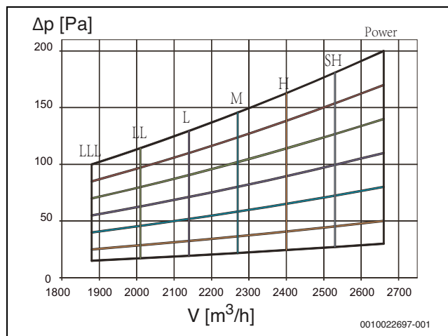
Рис. 29 AF-DH 160-1
