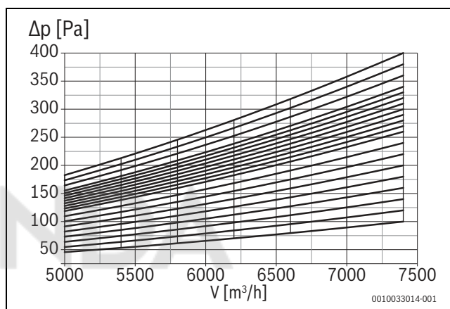
Рис. 34 AF-DH 560-1
