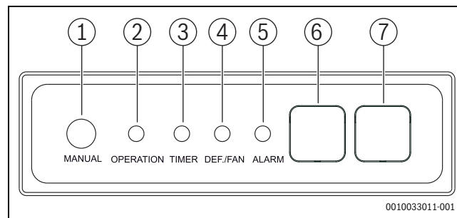
Рис. 47 Панель дисплея
