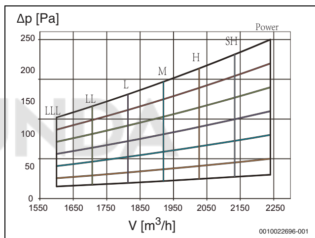
Рис. 28 AF-DH 140-1
