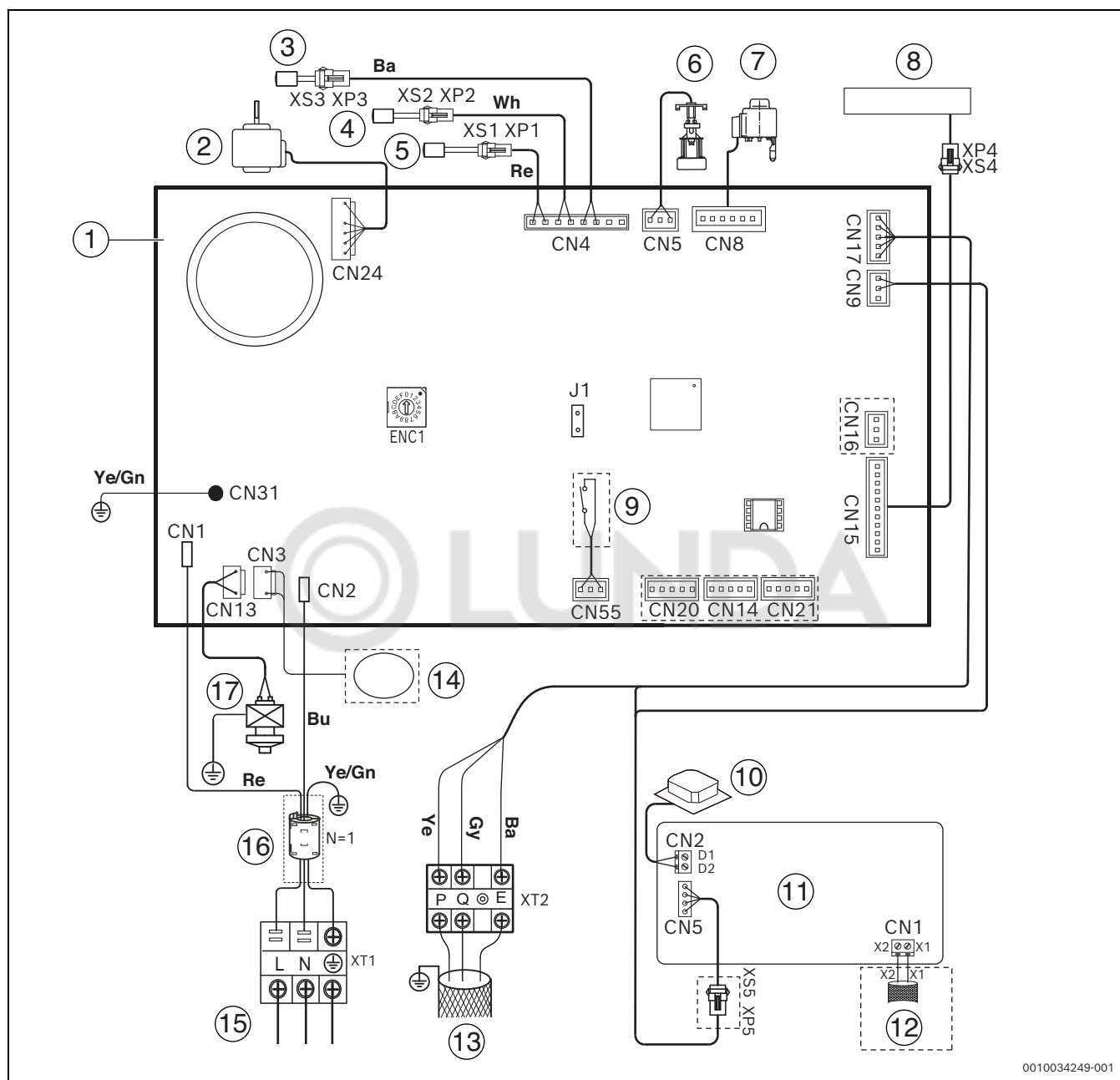
Рис. 49 Электропроводка
