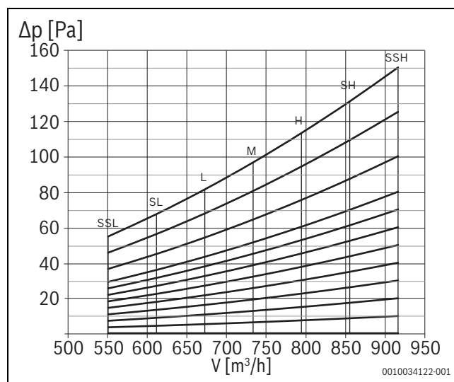
Рис. 28 Мощность вентилятора AF-DHS 45
