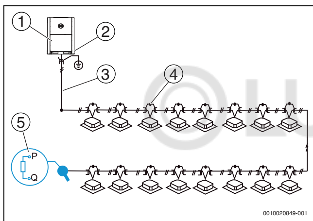
Рис. 39 Коммуникационная проводка внутренних и наружных блоков (PQE)
