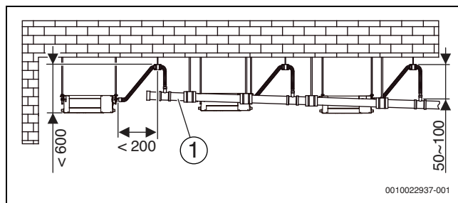
Рис. 19 Монтаж и расстояние между сливными трубами с водяным насосом [мм]
