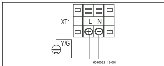
Рис. 35 Входное питание
