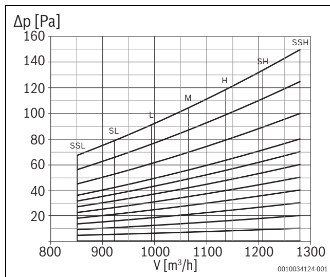
Рис. 30 Мощность вентилятора AF-DHS 71
