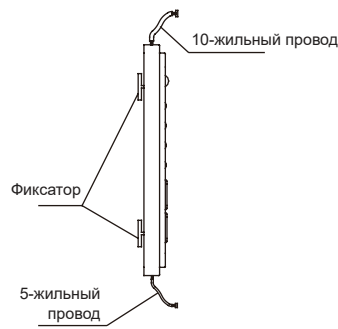
Рисунок 8.2 Плата индикации
