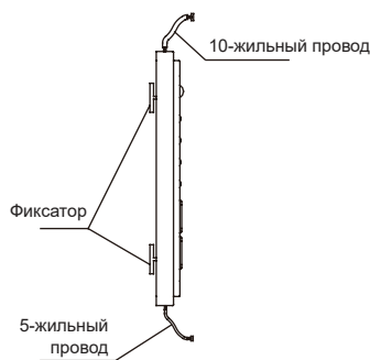
Рисунок 8.2 Плата индикации
