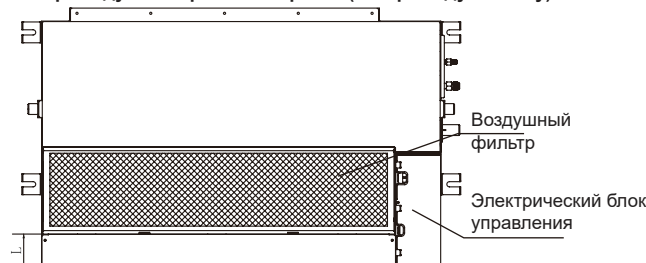
Размер воздухозаборного отверстия (забор воздуха снизу).
