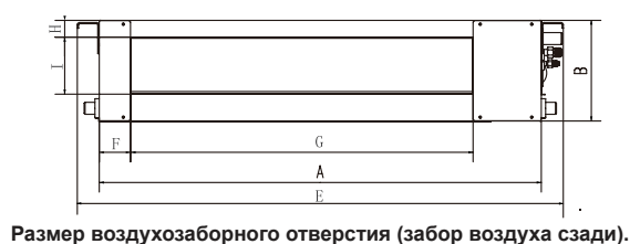
Размер воздухозаборного отверстия (забор воздуха сзади).
