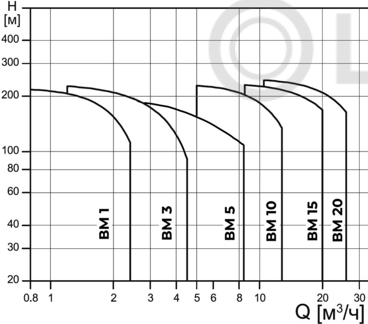
Диапазон характеристик насосов BM 1, 3, 5, 10, 15, 20
