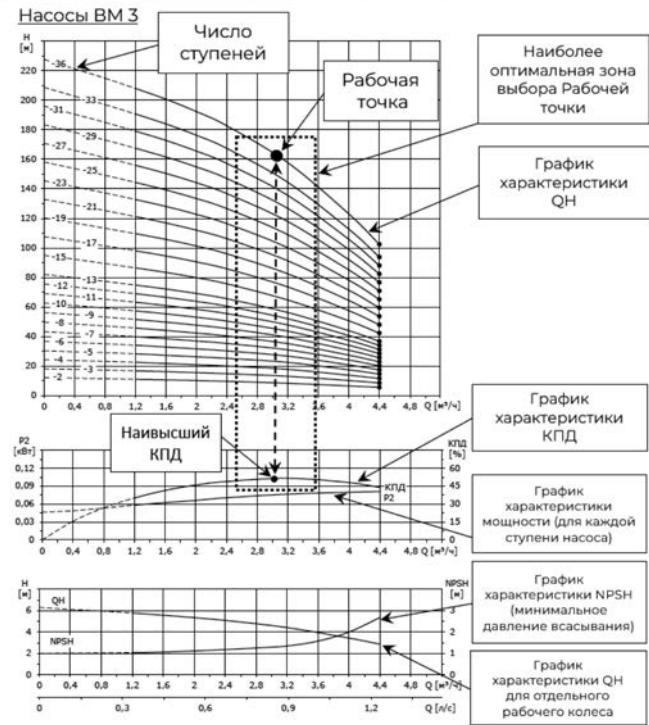
Расположение данных на диаграммах рабочих
