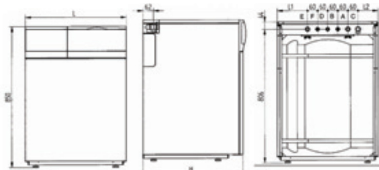
UB INOX 80 - 120 / SLIM UB INOX 80 - 120
