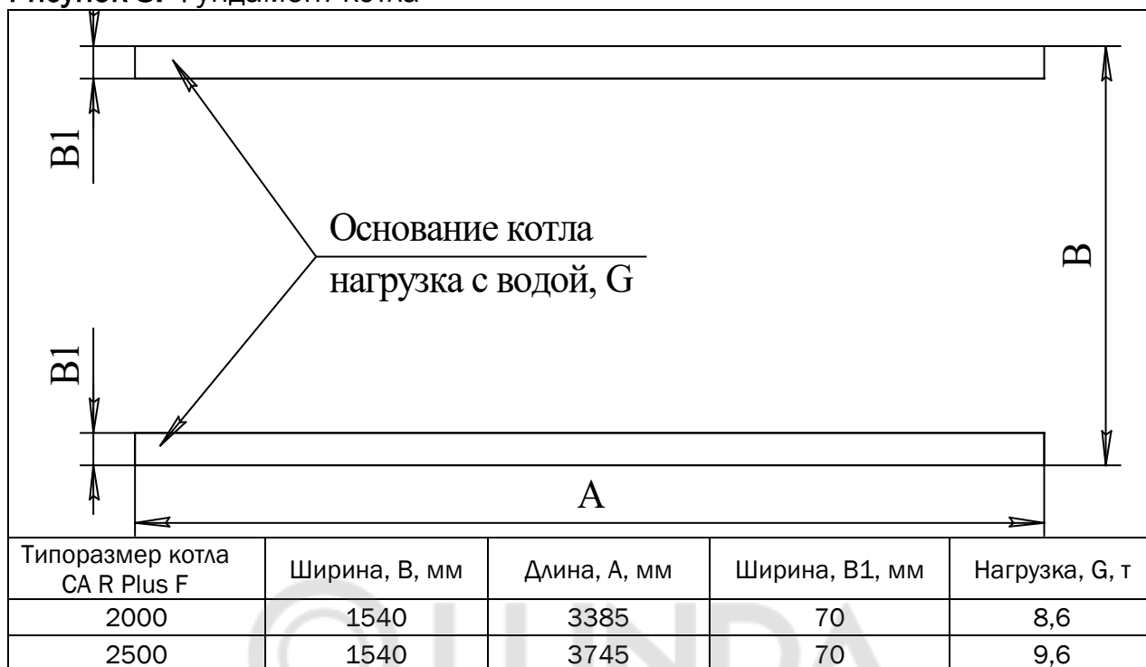
Рисунок 8. Фундамент котла
