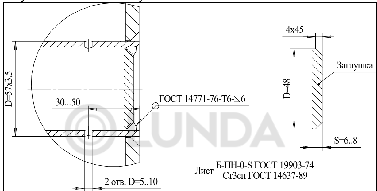
Рисунок 10. Установка заглушки
