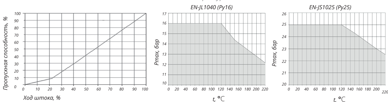
Зависимость давления, которое выдерживает корпус клапана, от температуры
