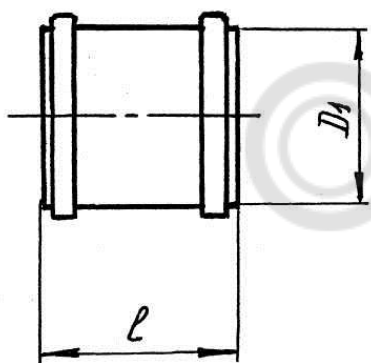
Муфта ремонтная
