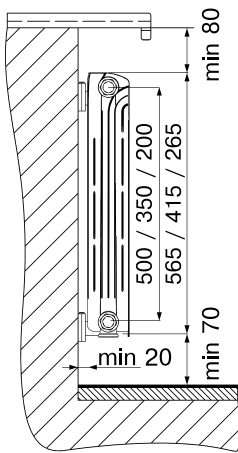
C – ширина секции
