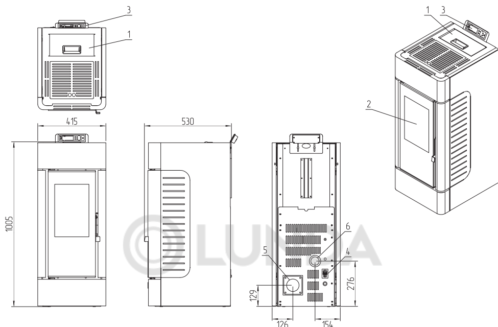
Рис.1 Устройство камина C12H22
