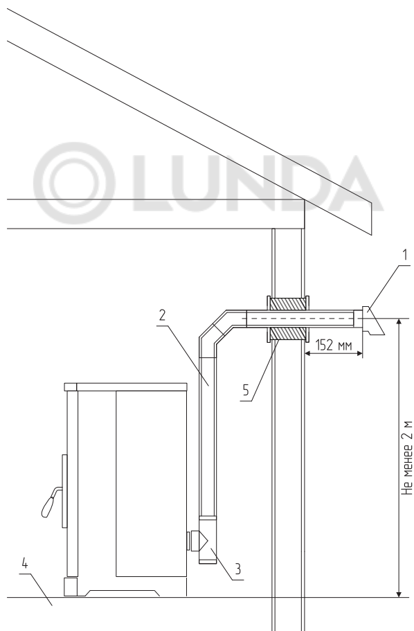
Рис.9 Подключение дымохода через стену
