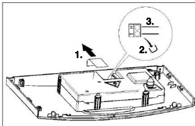
Рис. 21 Подключение регулятора
