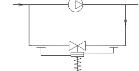
Установка регулятора на байпасе насоса
