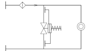
Установка регулятора на перемычке
