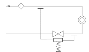
Установка регулятора на обратном трубопроводе
