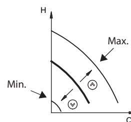
Рис. 14 Нерегулируемый режим
