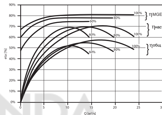
Рис. 3 КПД MGE электродвигателя, насоса и общий КПД E-насоса при частотах вращения 100%, 80% и 60% от максимальной скорости вращения вала насоса.
