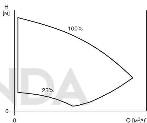
Рис. 26 Поле характеристик TPE серии 2000
