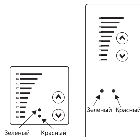
Рис. 24 Панели управления E-насоса
