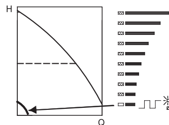
Рис. 21 Режим минимальной характеристики
