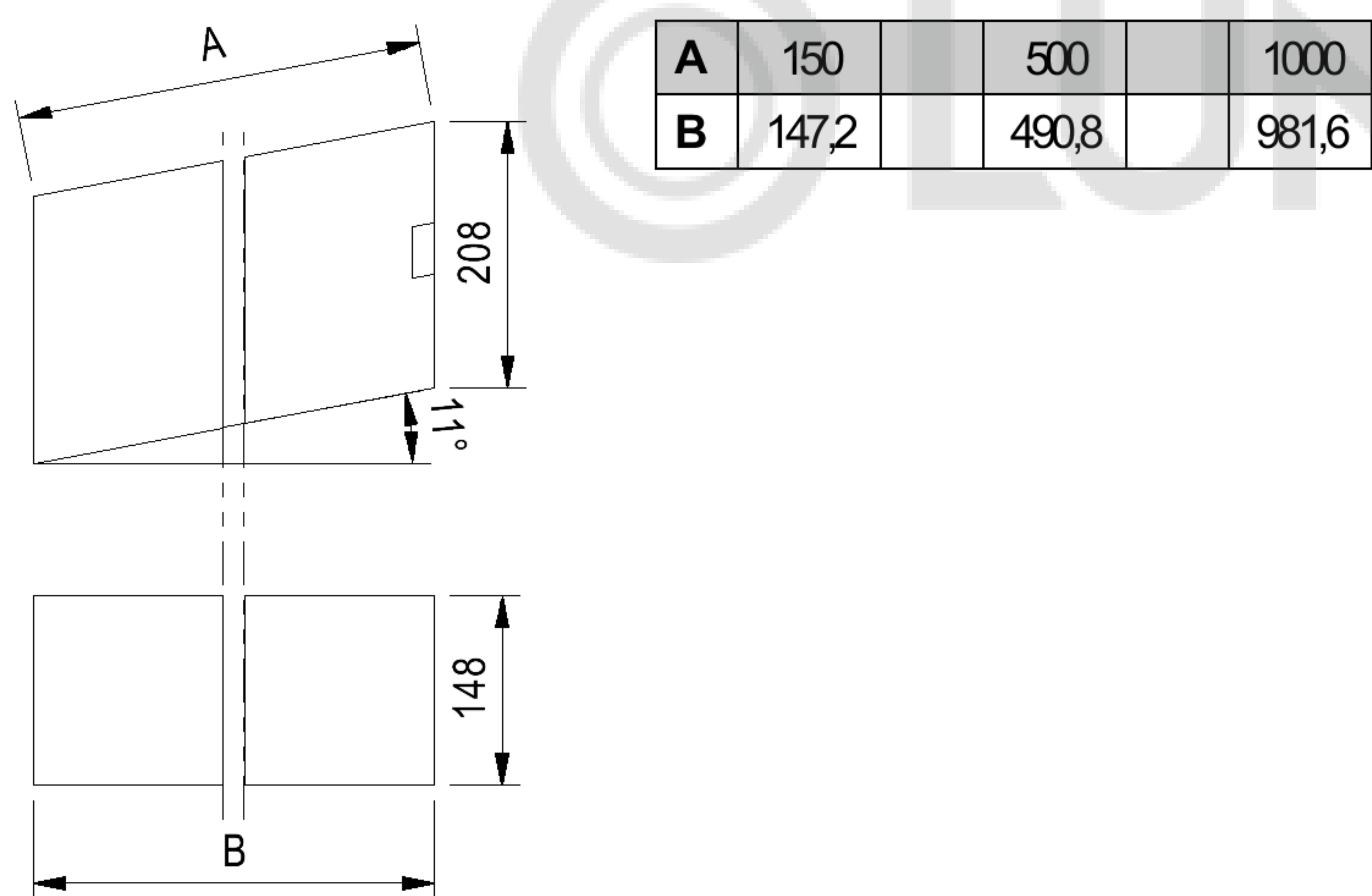
fu 11 Коробка-удлинение L=150/500/1000 мм для fu 09
