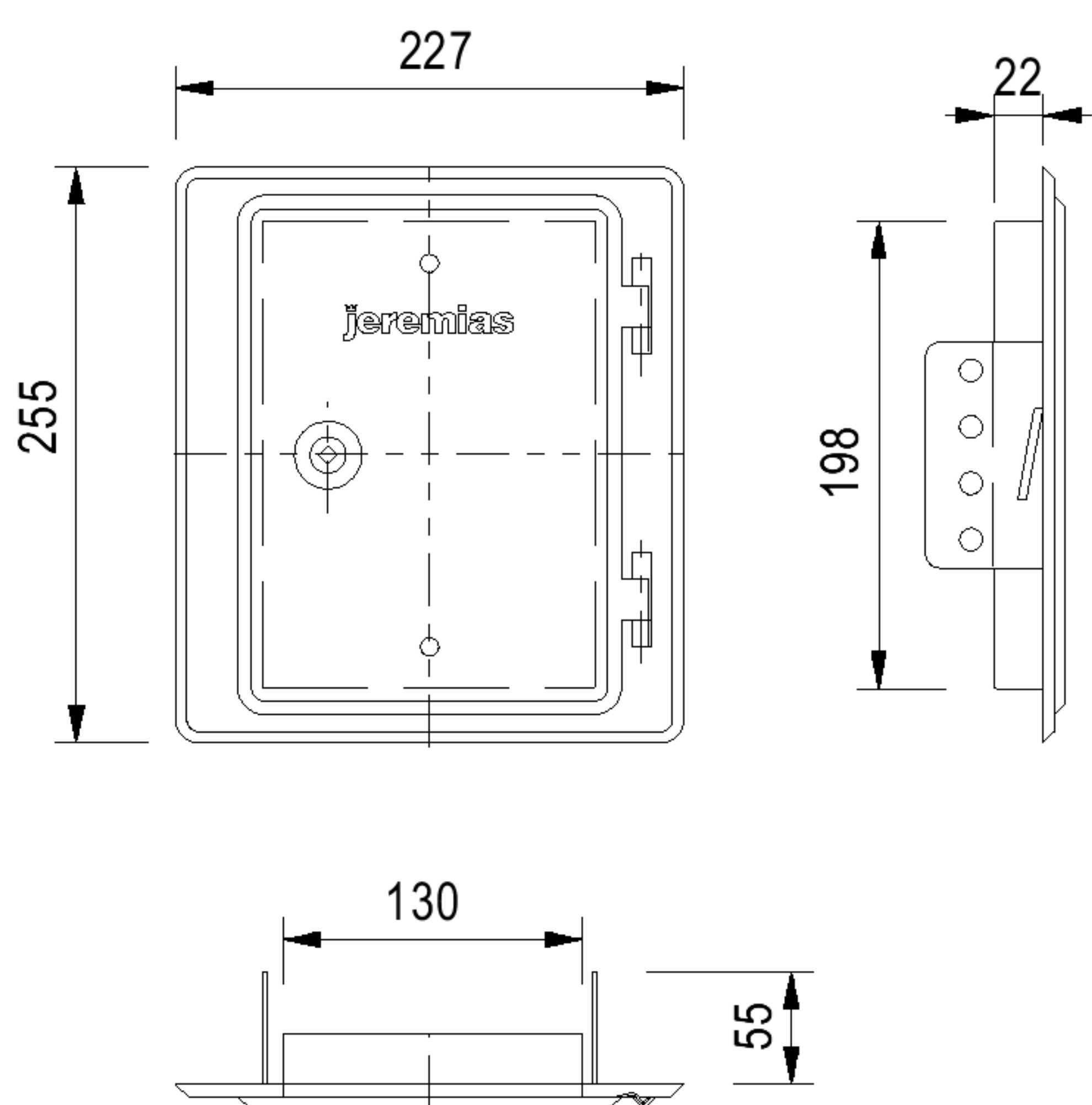
fu 13 Дверка ревизии 210 x 140 мм
