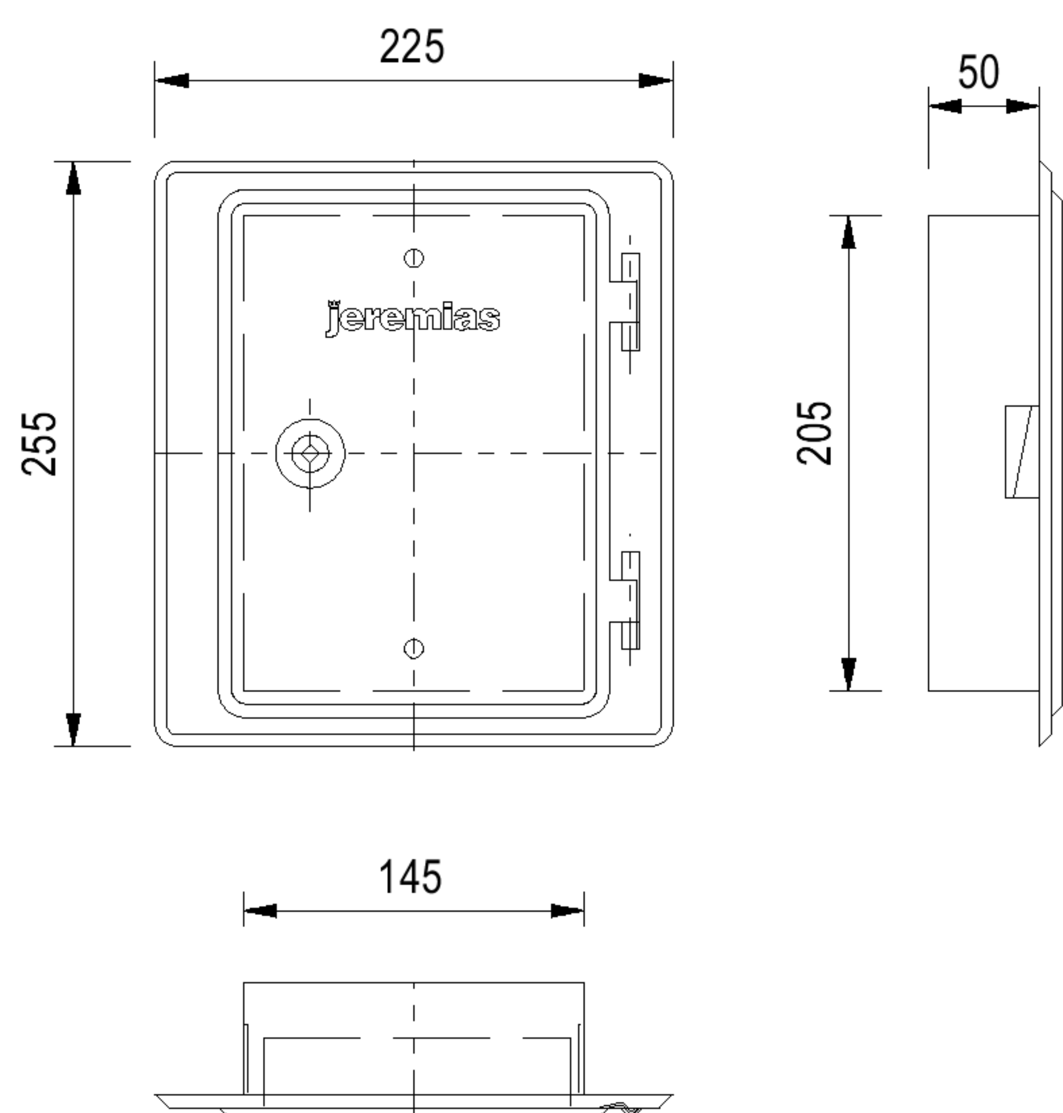
fu 09 Дверка ревизии 210 x 140 мм, вст авка 50 мм
