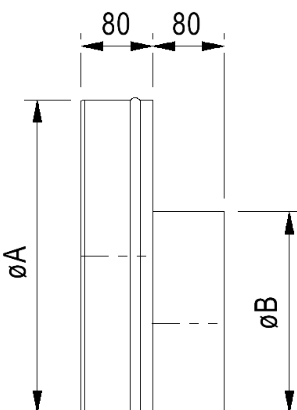
fu 124 Присоединит ельный пат рубок переходной, эксцент рический, вст авной
