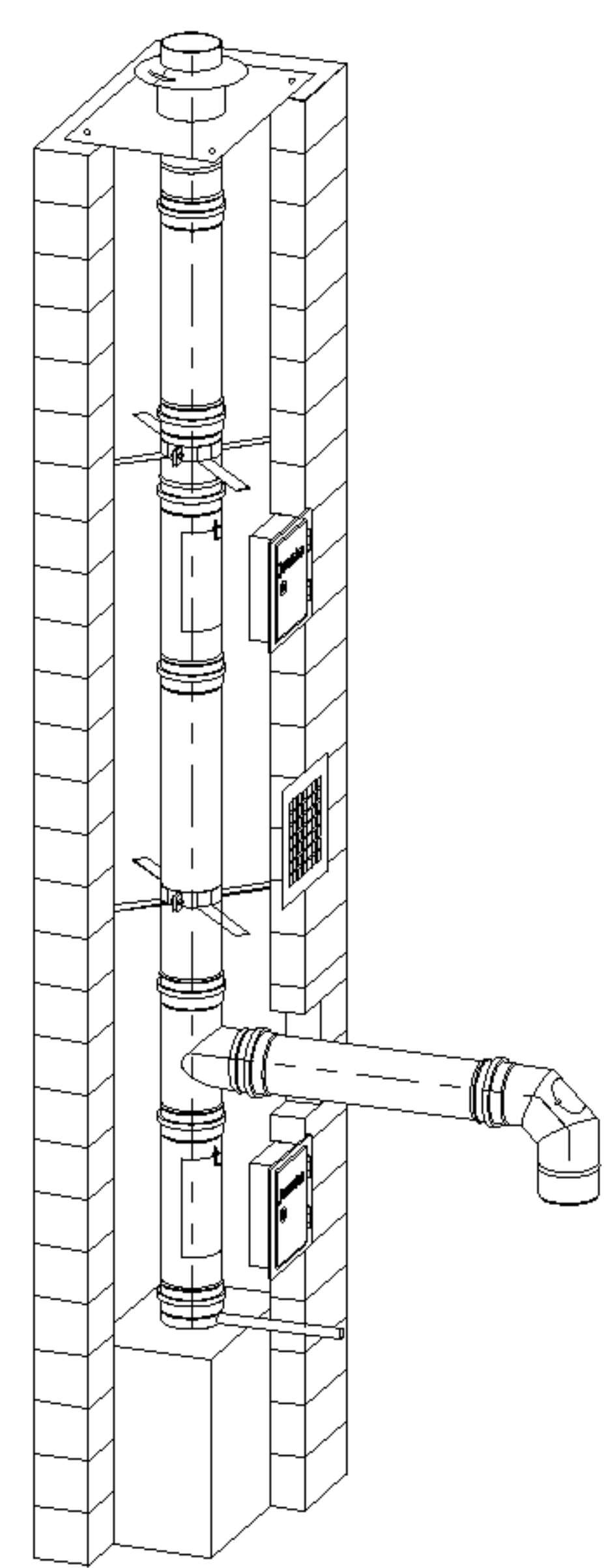
Рис. 3: стандартное устройство
