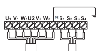
Подключение звезда/треугольник
