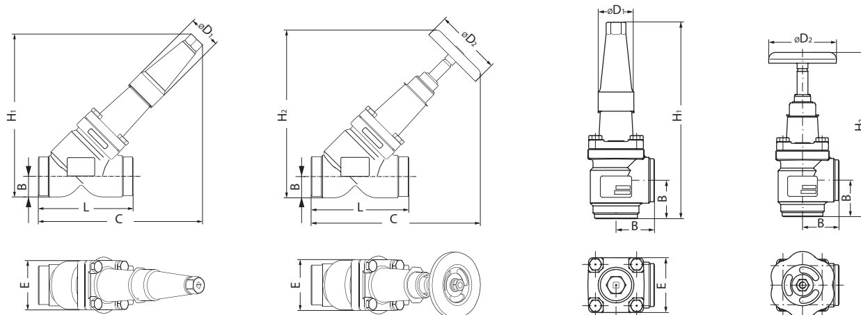
Прямые запорные клапаны REG XXX STR
