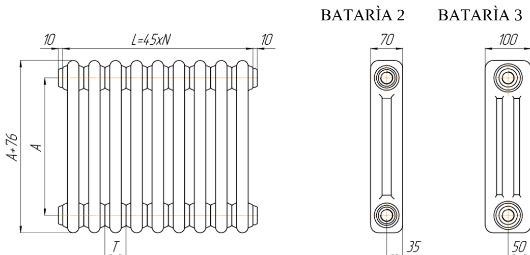
Рис. 1. Т – шаг (45мм), N – количество секций.
