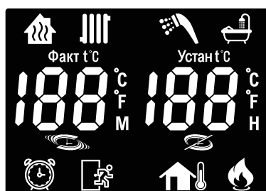
Рисунок 8. Дисплей пульта управления NCTR-60R.
