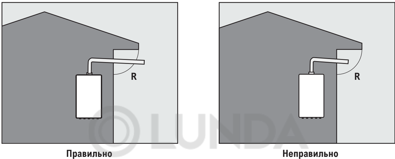
Рисунок 10. Зона повышенного давления воздуха.
