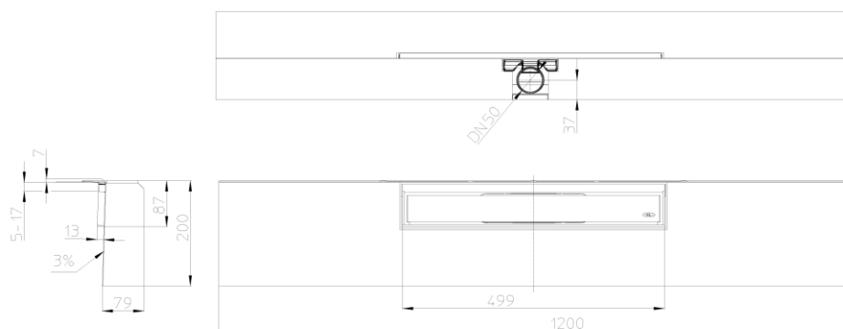
Рис. 1. Корпус лотка HL531
