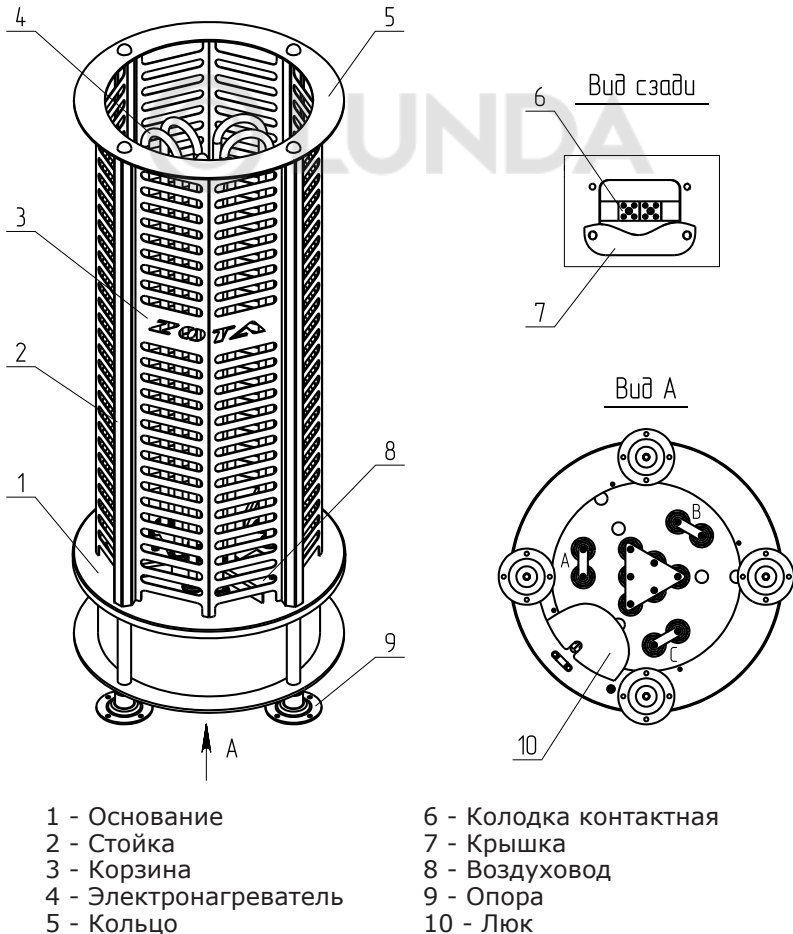
Рис.1 Конструкция электрокаменки
