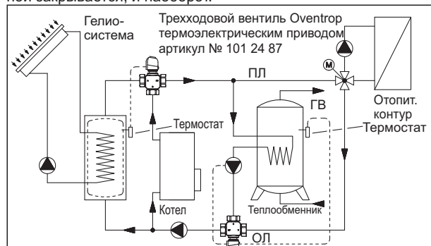
Трехходовой вентиль Oventrop с термоэлектрическим приводом со вспомогат. выключателем артикул № 101 24 87
