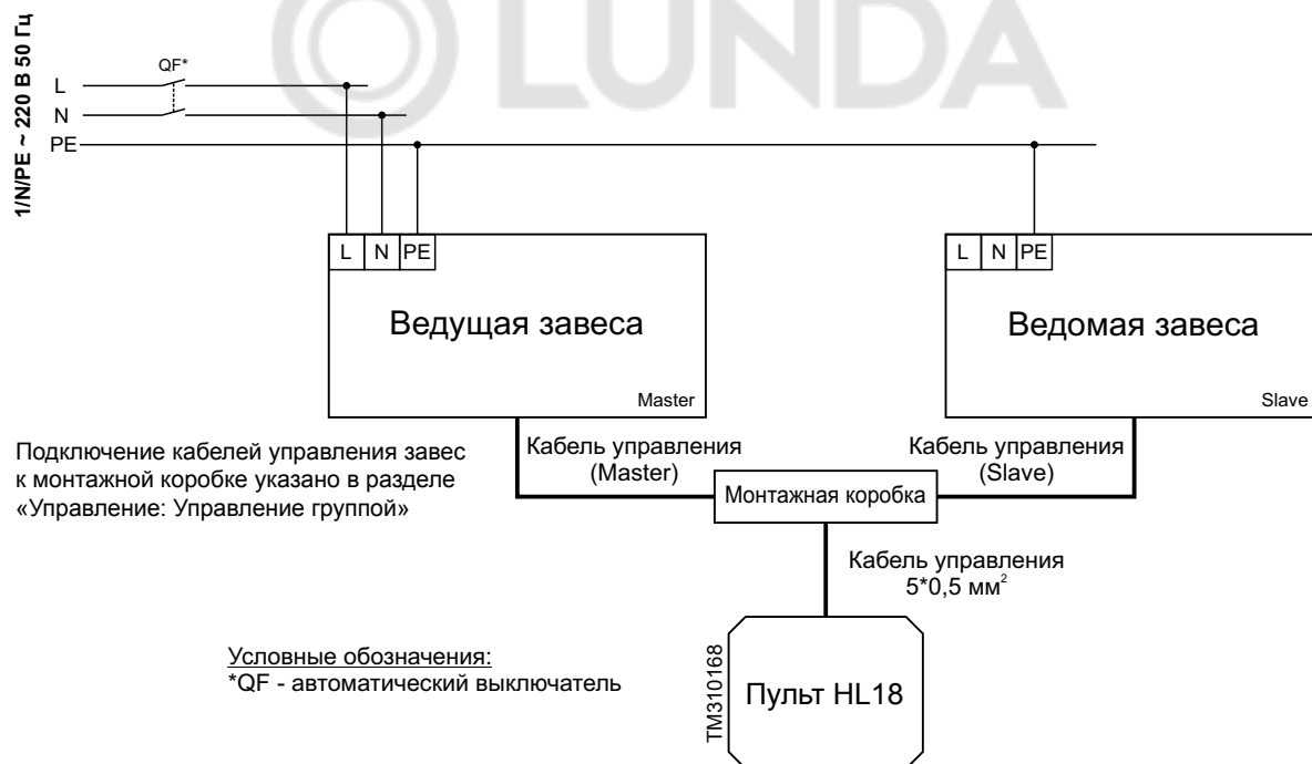
Схема подключения группы завес к однофазной сети переменного тока с напряжением ~220 (230) В
