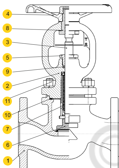
Исполнение 01,11
