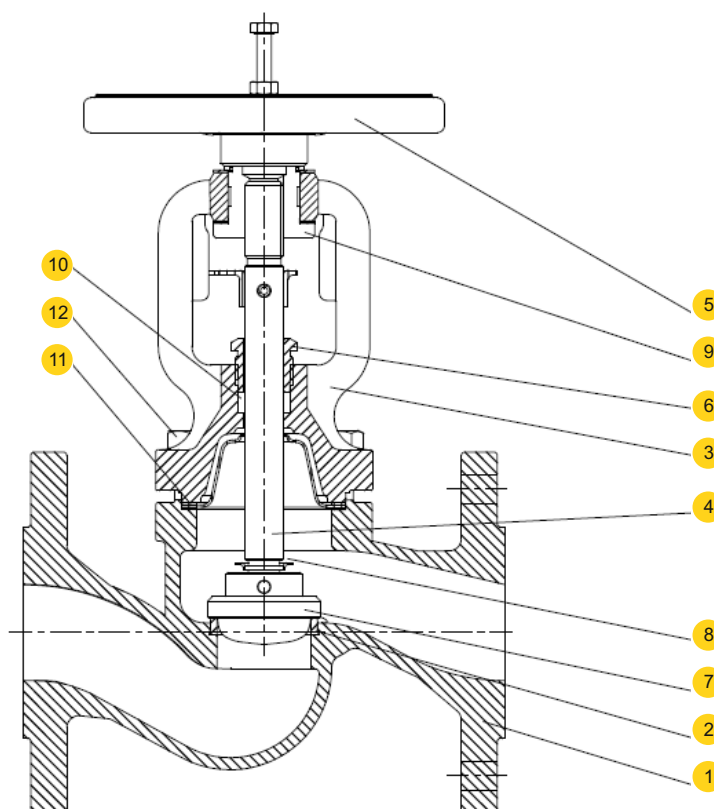
Исполнение 71
