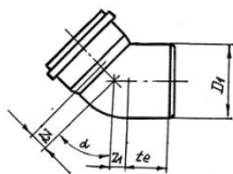
Рисунок 7. Отвод
