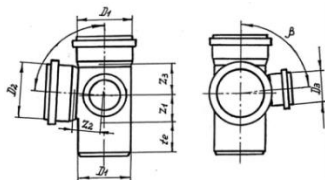
Рис 5.2. Крестовина двухплоскостная(левое исполнение)
