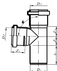
Рисунок 13. Тройники
