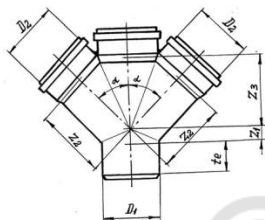
Рис 4. Крестовина одноплоскостная
