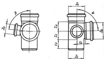
Рис 5.1. Крестовина двухплоскостная
