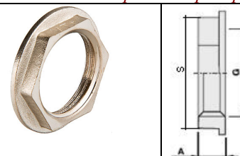
VTr. 655 Контргайка с ребордой В
