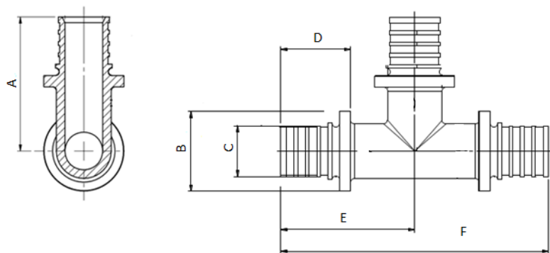
Тройник редукционный
