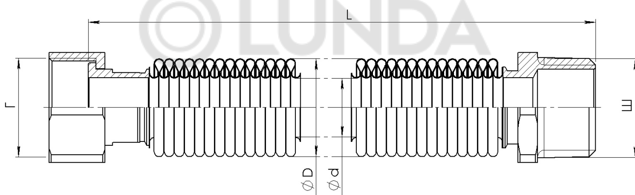
Рисунок 6. Шланг универсальный для воды и газа раздвижной.
