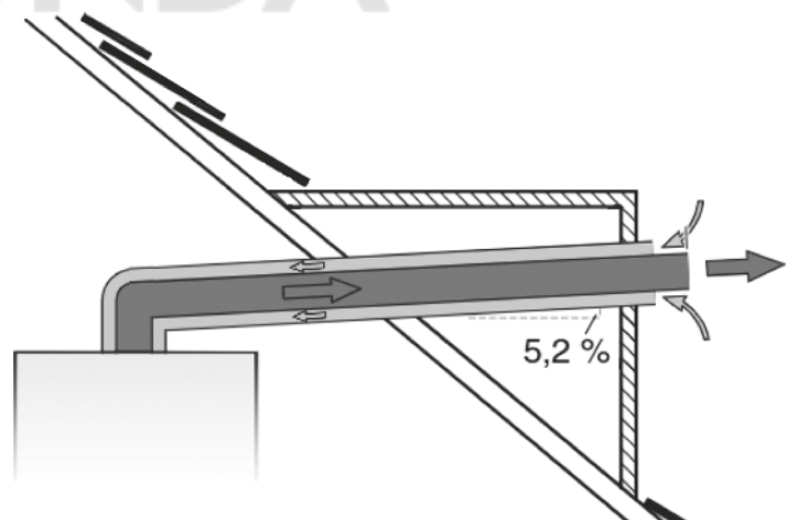
Рис. 33. Угол наклона дымохода.
