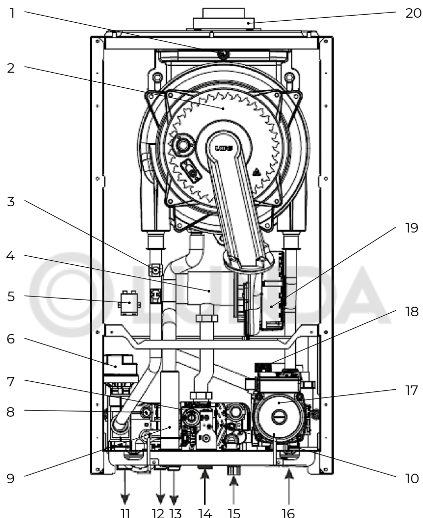
Рис. 3. Общая схема М30 36 С.
