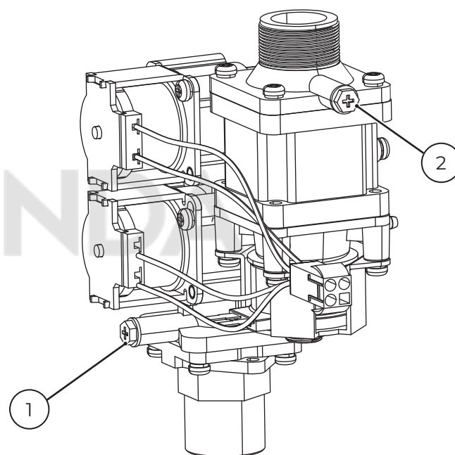
Рис. 25. Газовый клапан.
