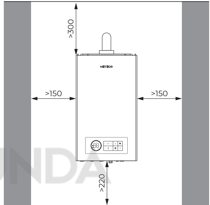
Рис. 29. Рекомендуемые расстояния для монтажа.
