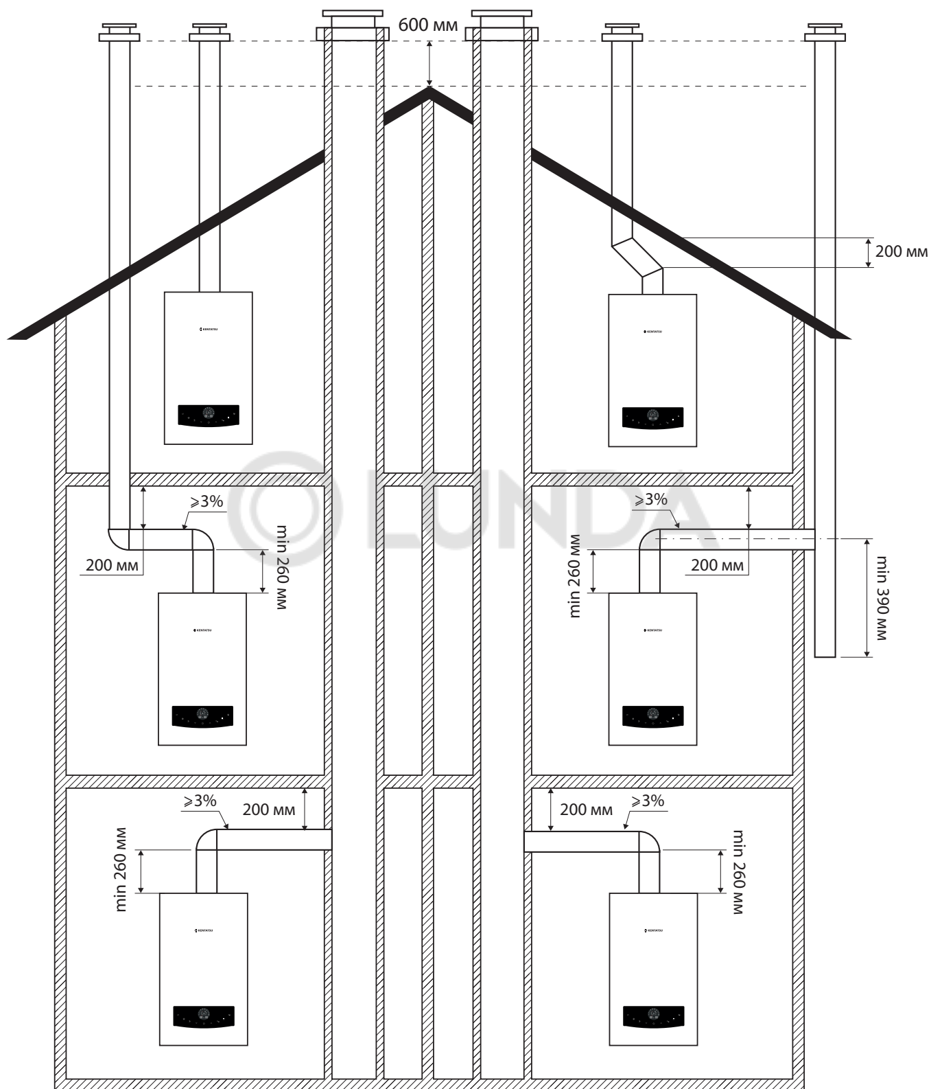
Примеры установки дымоходов и воздуховодов
