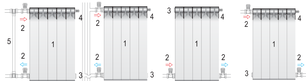
Диагональное (рекомендуется для получения максимальной теплоотдачи)
