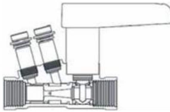
Рис. 10 конструкция клапана Ballorex Venturi FODRV
