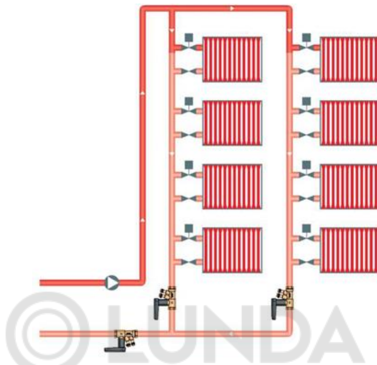
Рис. 2 Однотрубная стояковая система отопления
