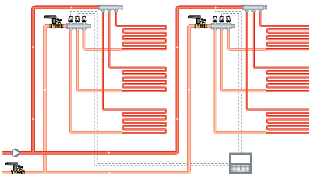
Рис. 5 Система отопления теплыми полами
