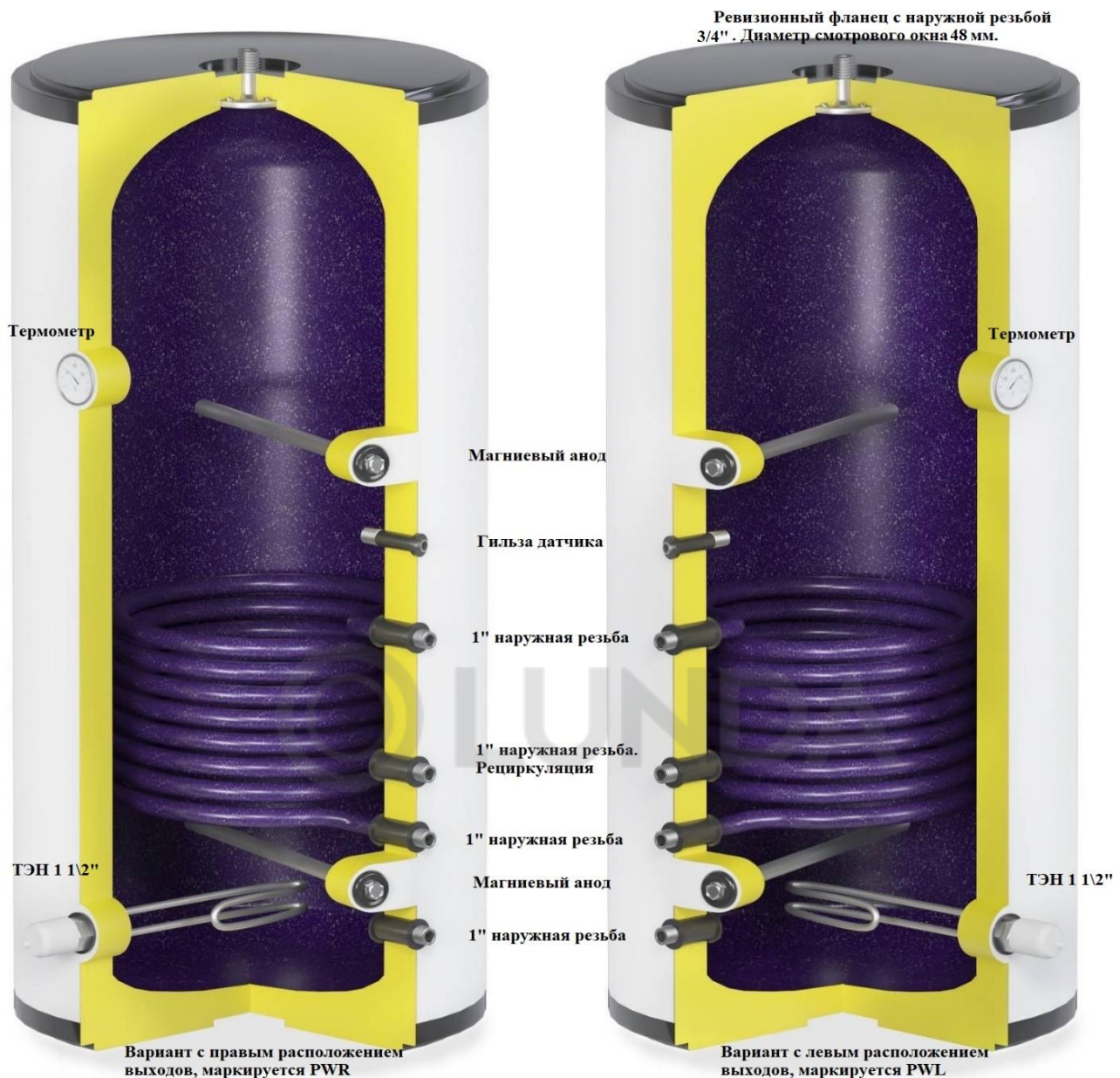
PWR- с правым подключением
