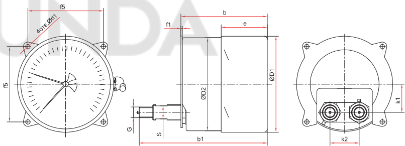
Эксцентрическое присоединение с задним фланцем (ТМ2ж)
