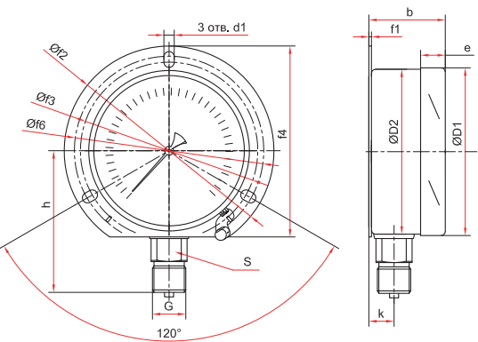
Радиальное присоединение с задним фланцем (ТМж)
