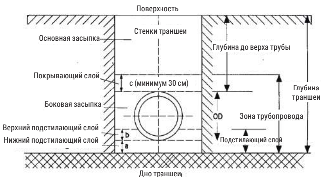
РИС. 3. УСТРОЙСТВО ТРАНШЕИ
