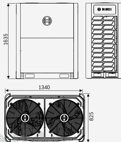
Размеры (в мм) блоков серии Air Flux 6300A (C) мощностью 40–50 кВт
