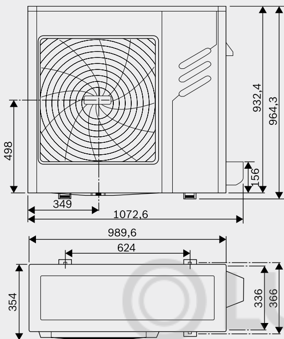
Размеры (в мм) блоков серии MDCI мощностью до 10 кВт
