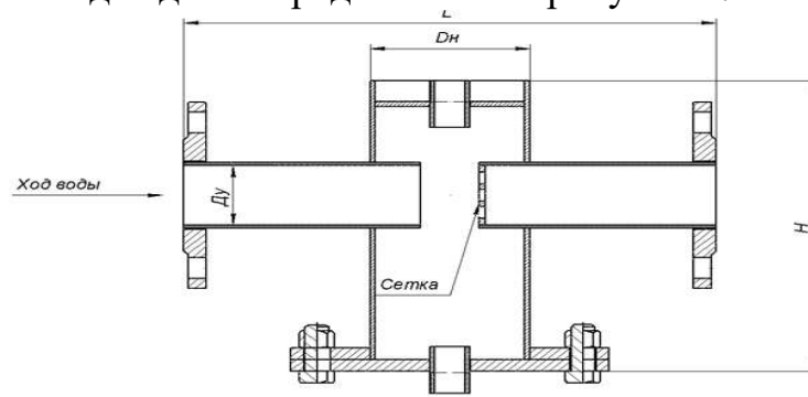
Рисунок 1 – Внешний вид изделия
