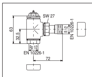
Размеры
