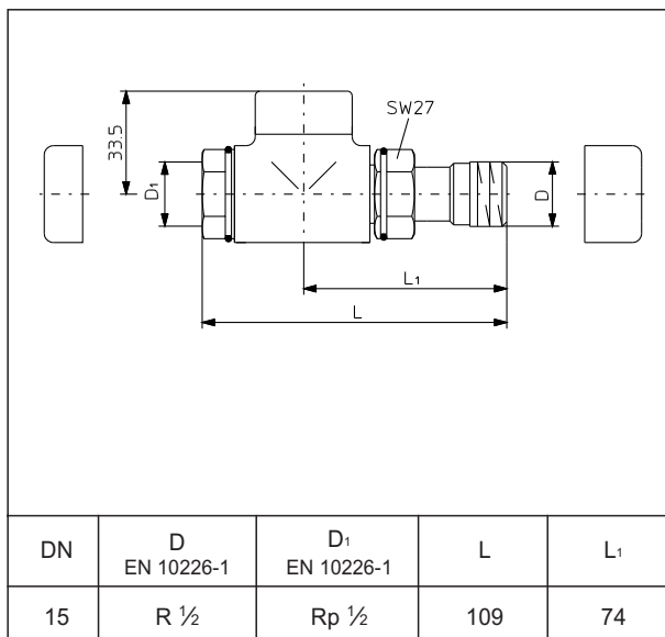
Размеры
