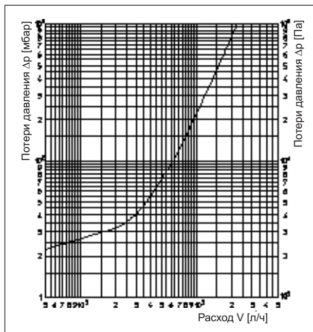
Диаграмма расходов „Regumat F-130“/F-180/FR-180
