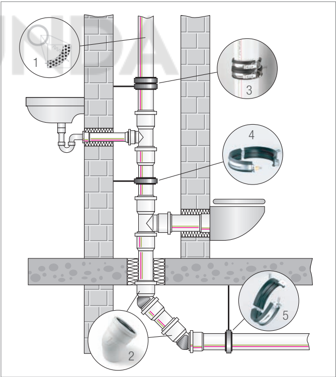
Рис. 4-1 Минимизация шума
