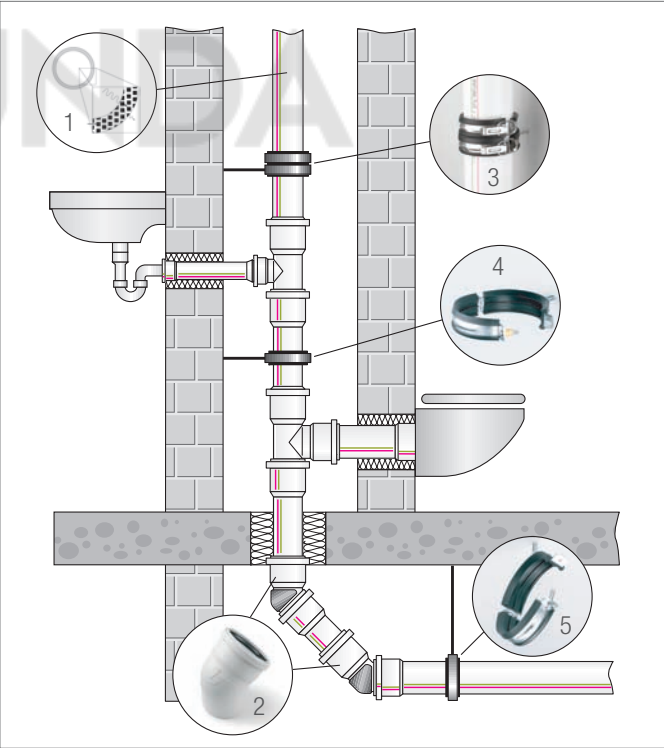
Рис. 4-1 Минимизация шума
