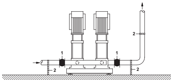
Рис. 3 Крепление трубопровода
