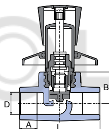
Вентиль под штукатурку проходной с металлической рукояткой
